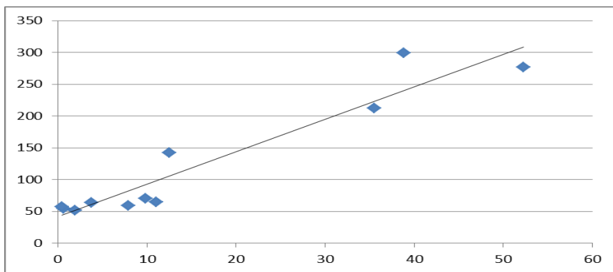
Рис. 1. Лінія тренду
