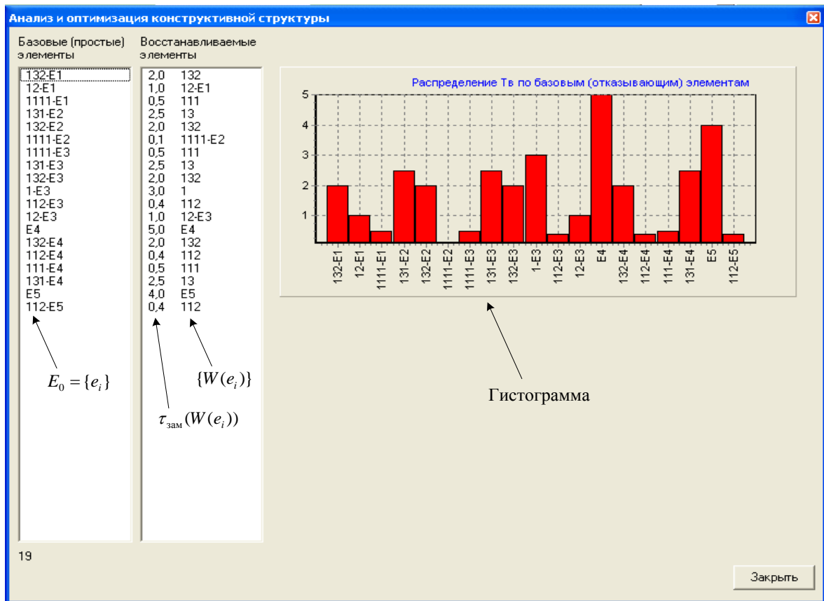
Рис. 4. Вигляд екрана ПК після виконання розрахунків для вихідної конструкції
