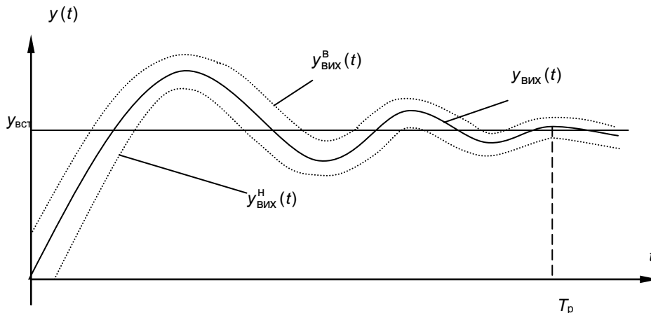
Рис. 1. Граничні криві функції працездатності аналогового пристрою в динамічному режимі
