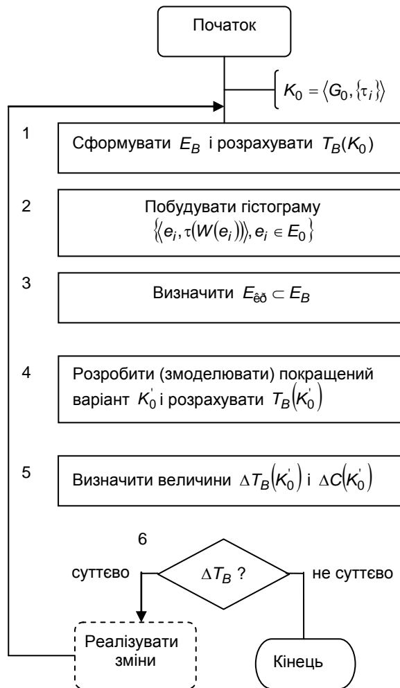
Рис. 2. Алгоритм оптимізації конструкції за критерієм
