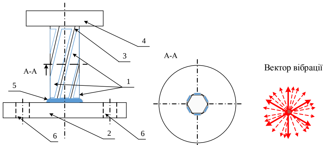
Рисунок 1. Вібродатчик на балці шестигранного типу з симетричного тензопреобразователь: 1-тензопреобразователь; 2-підставу для кріплення отворами 6; 3-шестигранна балка вібратора; 4 - балансир; 5 - місце зварювання
