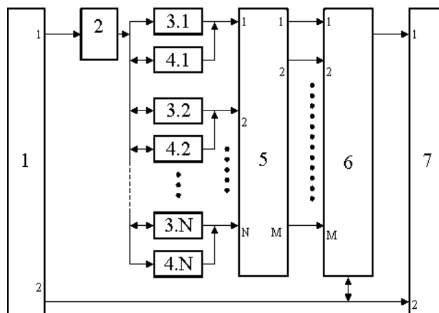
Рис. 1. Комбінований регулятор напруги змінного струму
