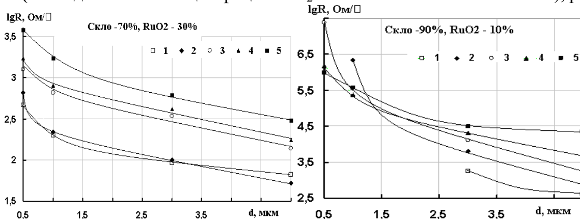
Рис.1. Залежність питомого поверхневого опору R_s , \Omega/\square від розмірів часток скла і температури відпалювання (1 – 500^\circ\text{C} , 2 – 600^\circ\text{C} , 3 – 700^\circ\text{C} , 4 – 800^\circ\text{C} , 5 – 900^\circ\text{C} )
