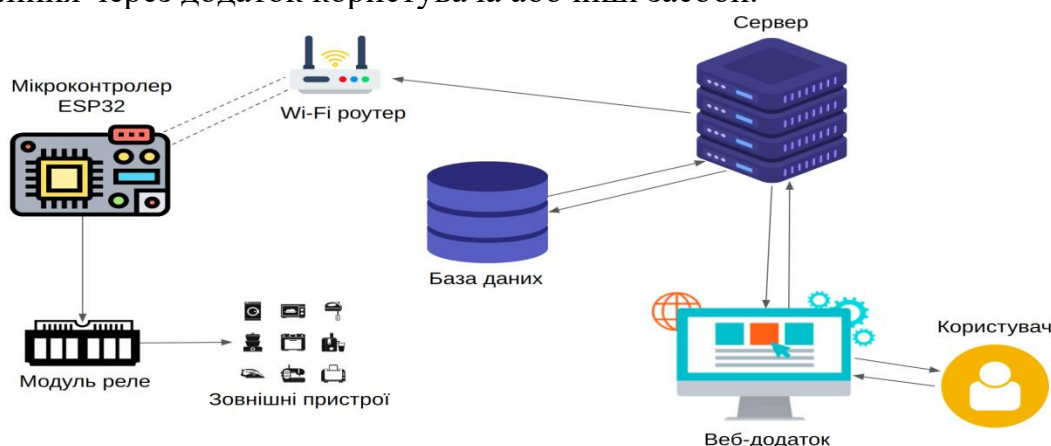
Рисунок – 1. Структурна схема взаємодії складових частин мережевої системи віддаленого управління пристроями
