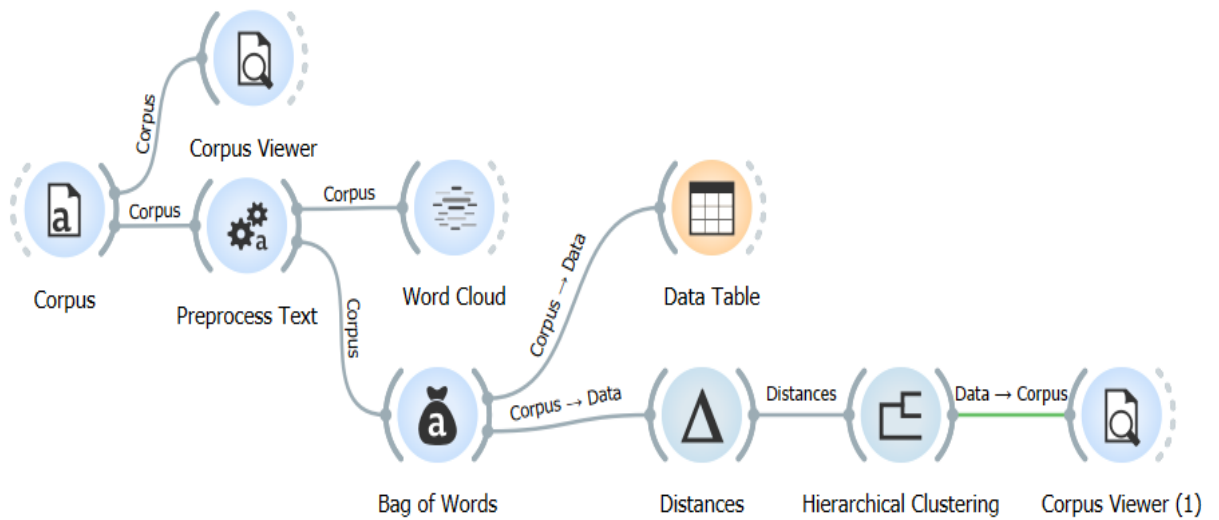
Рисунок 2. Схема ієрархічної кластеризації у середовищі «Orange».
