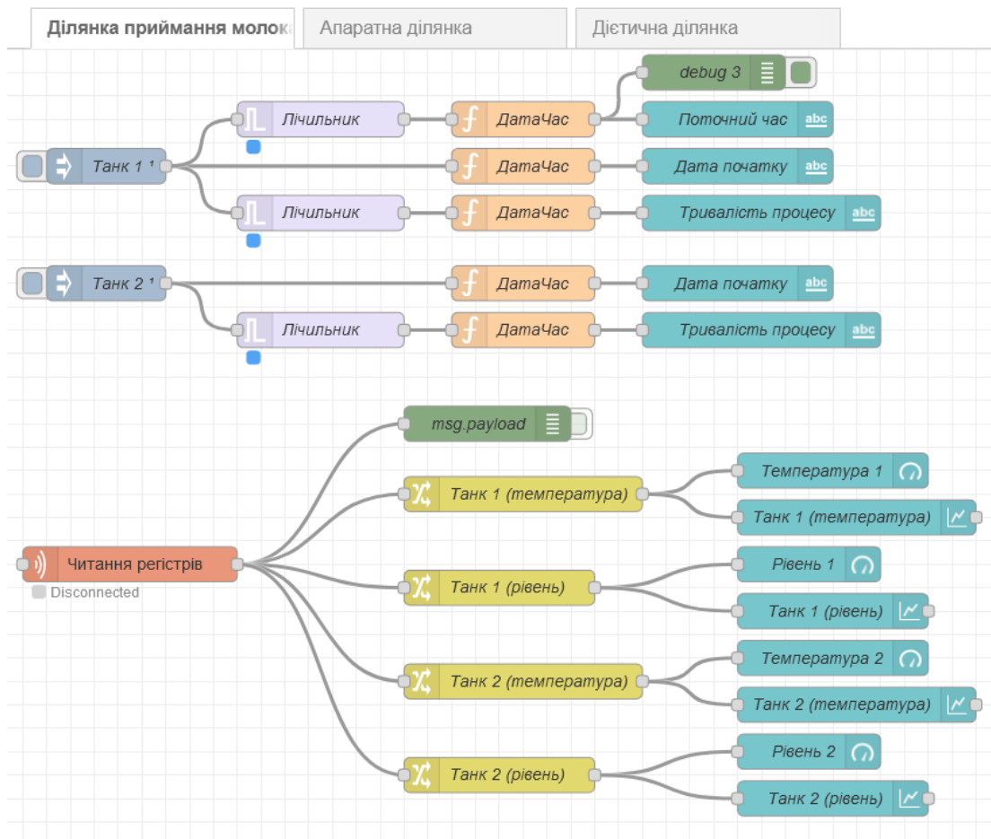
Рисунок – 1. Цифровий двійник ділянки приймання молока
