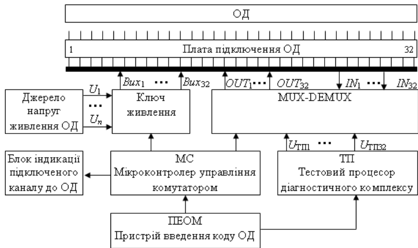
Рисунок – 1. Структурна схема керованого комутатора.
